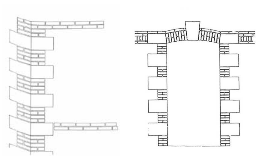
Chaînage d'angle
